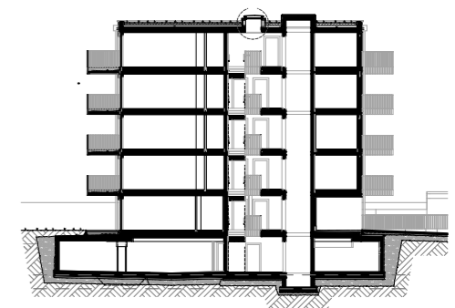
Schema Querschnitt
