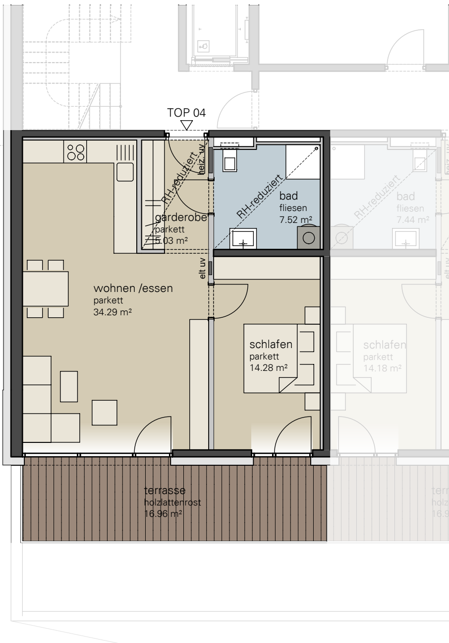
Wohnungsplan
