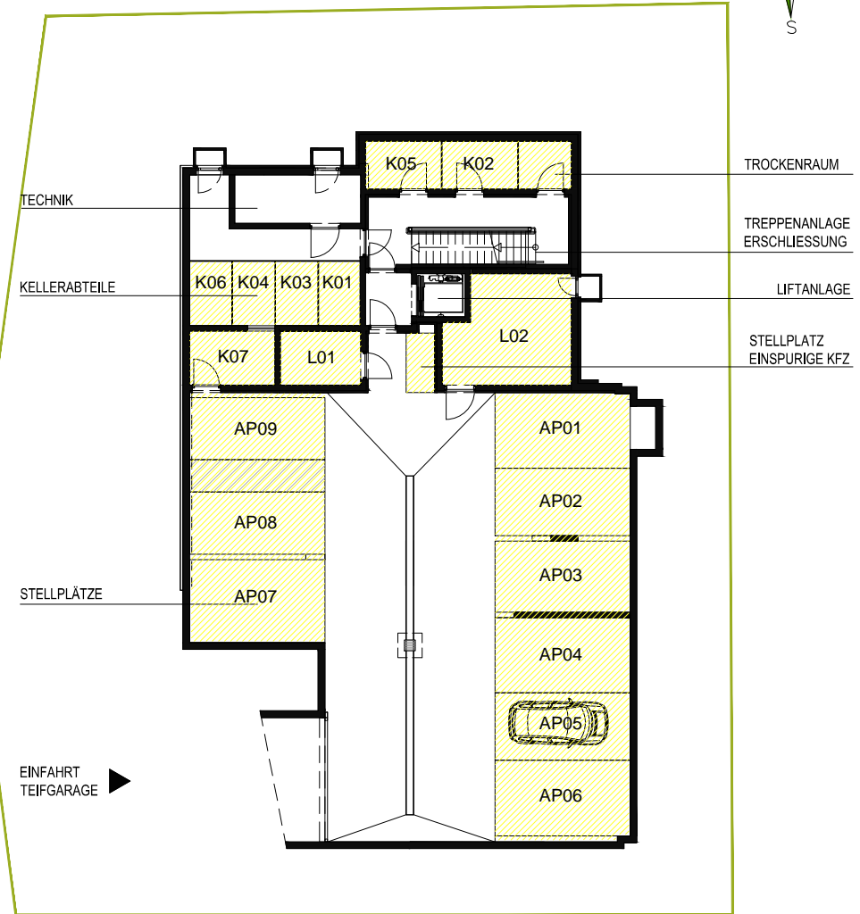
UNTERGESCHOSS
