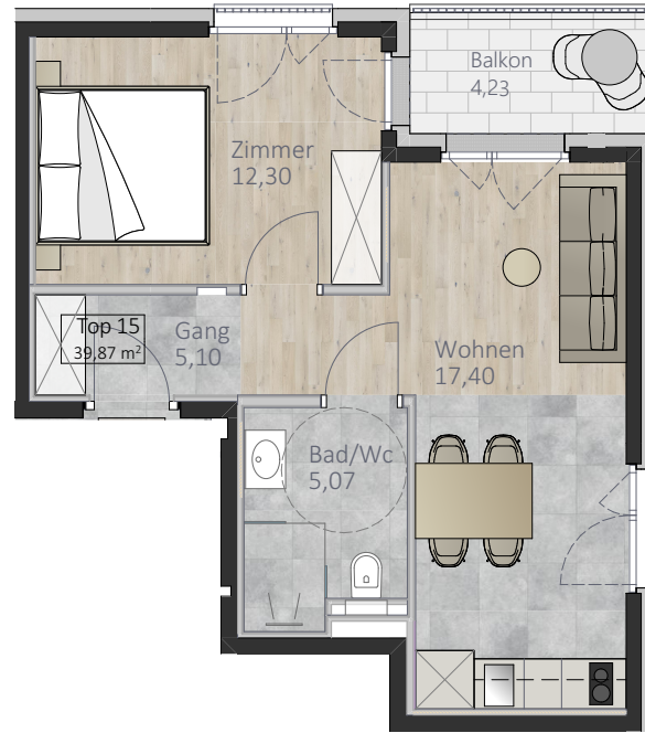
3. 3. Obergeschoss 1:100
