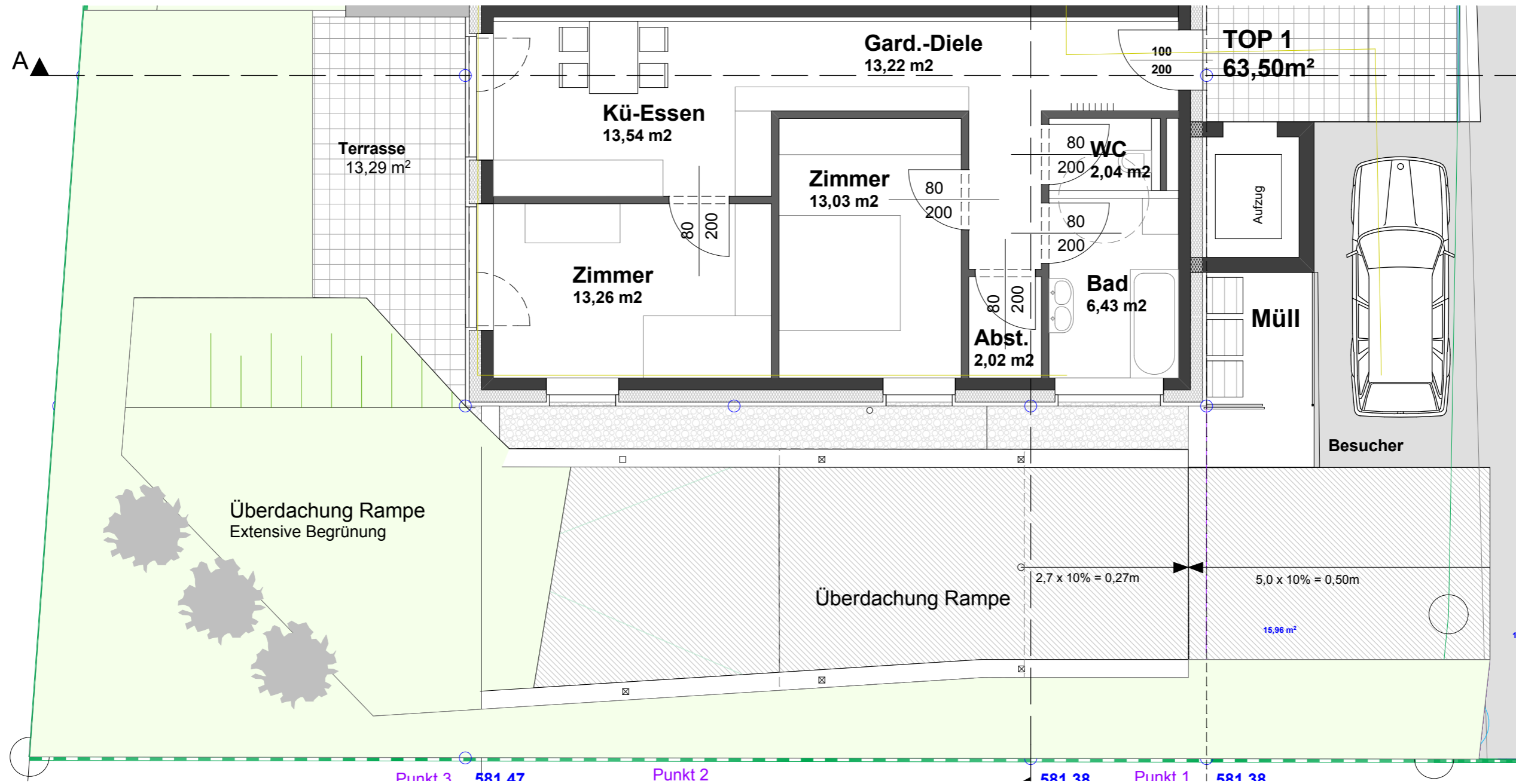
TOP 1 GRUNDRISS 1:75
