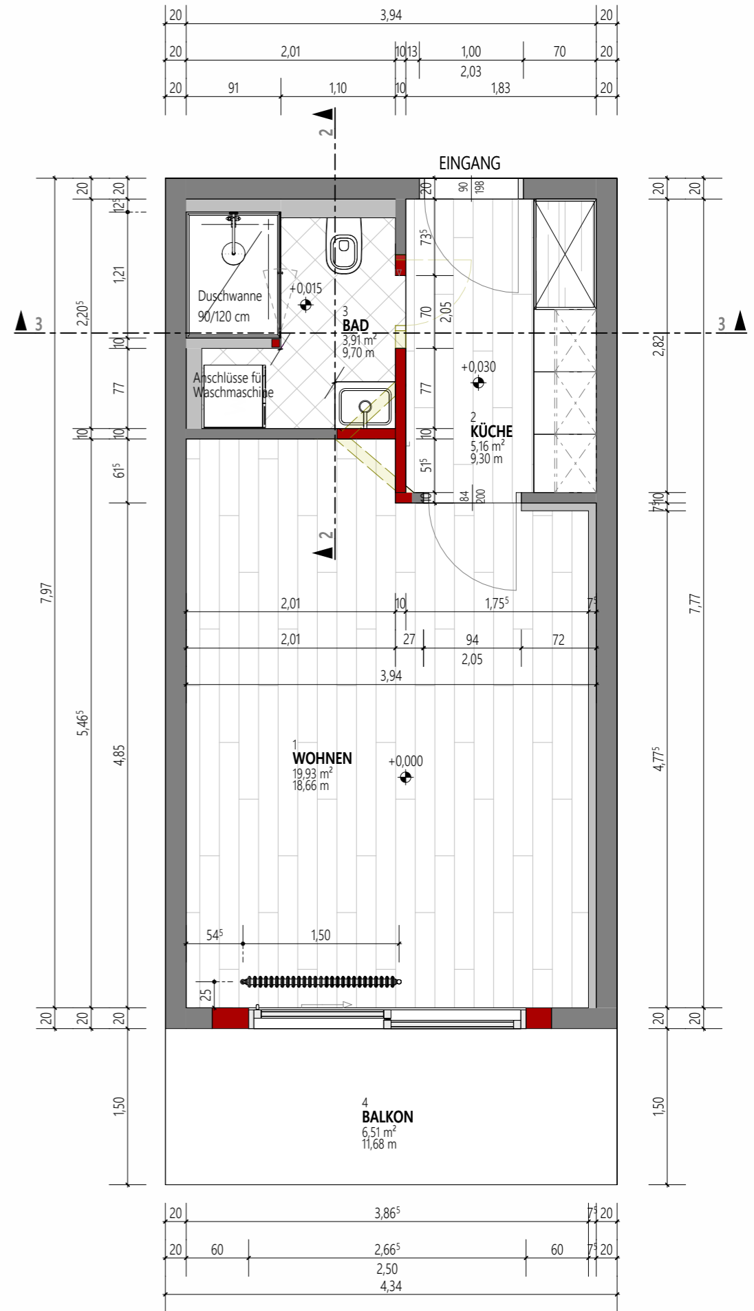
GRUNDRISS
