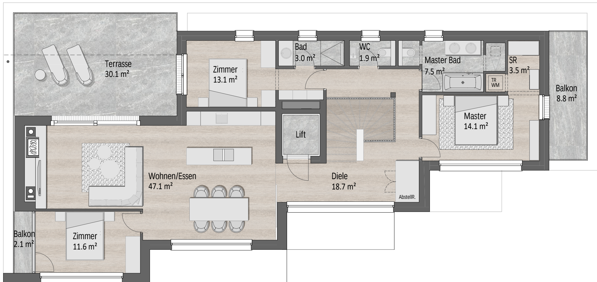
Variante 4-Zimmer Wohnung Grundriss Top 06, Alte Schmitte Fulpmes, Penthouse Wohnung, M 1:100
