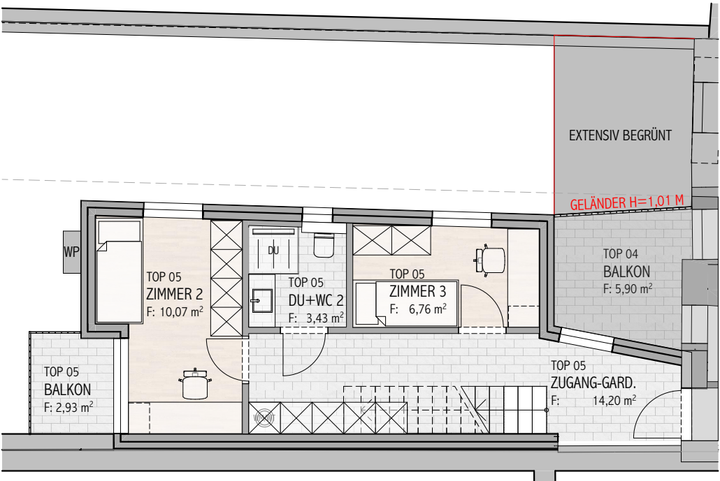
1 OBERGESCHOSS 1:100
