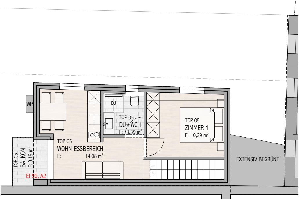
2 OBERGESCHOSS 1:100
