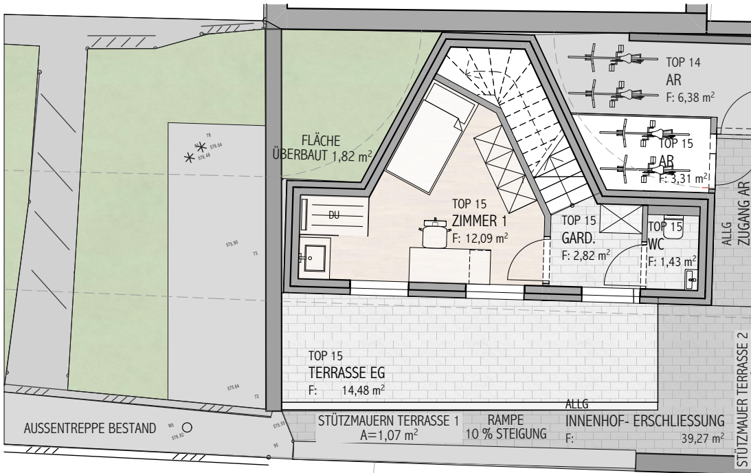
ERDGESCHOSS
