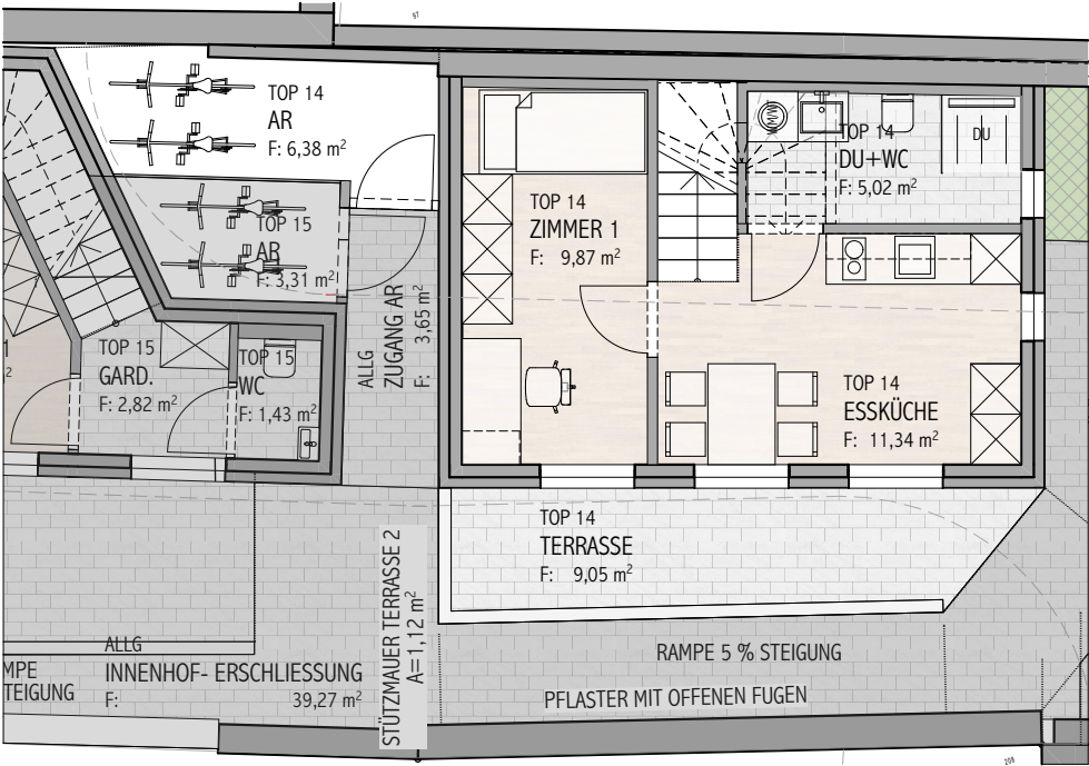
ERDGESCHOSS 1:100
