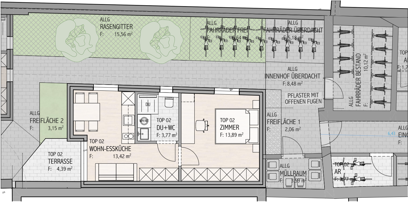
ERDGESCHOSS
