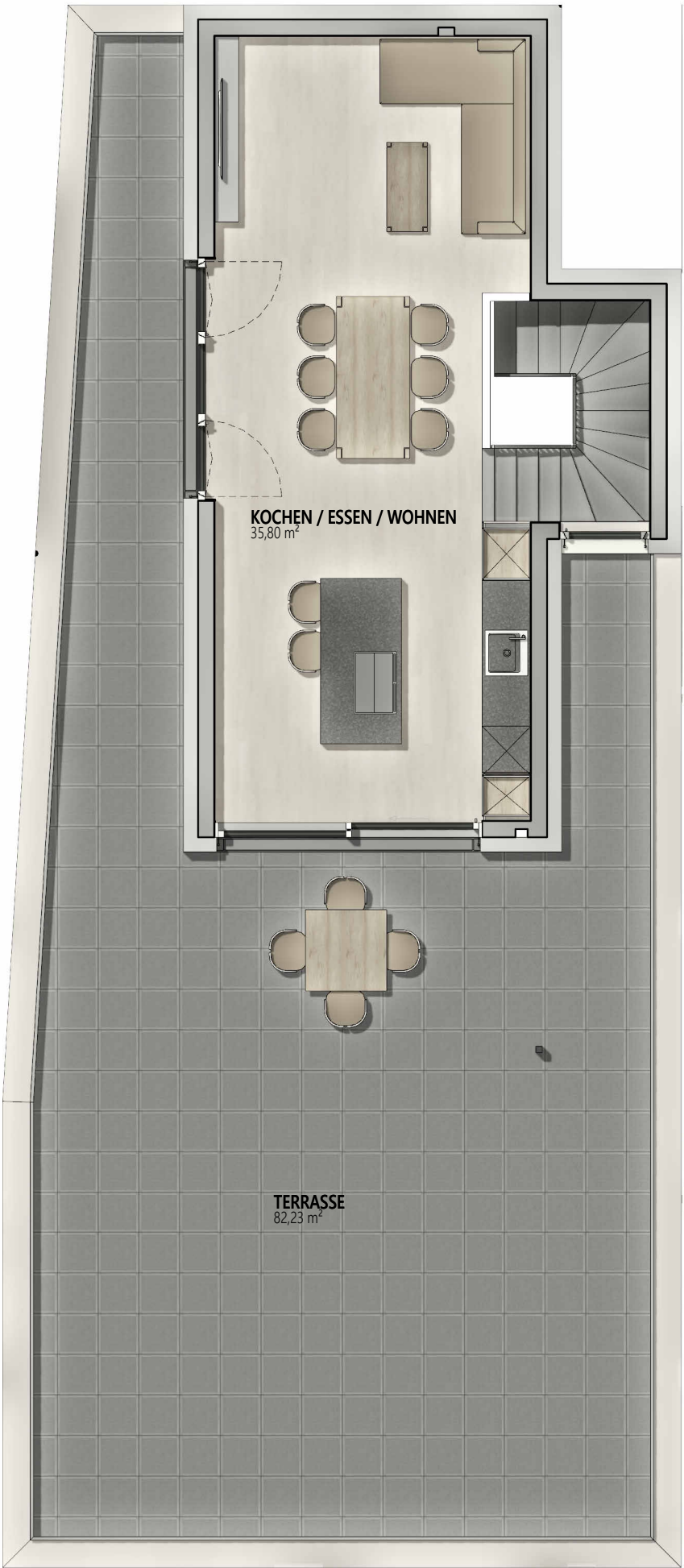
+2. Obergeschoss
