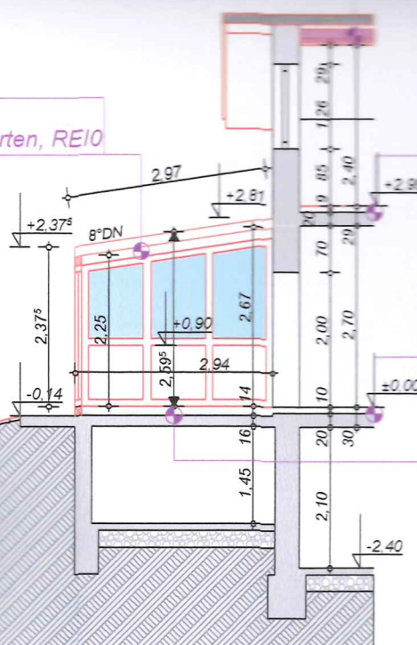
Schnitt 2-2
