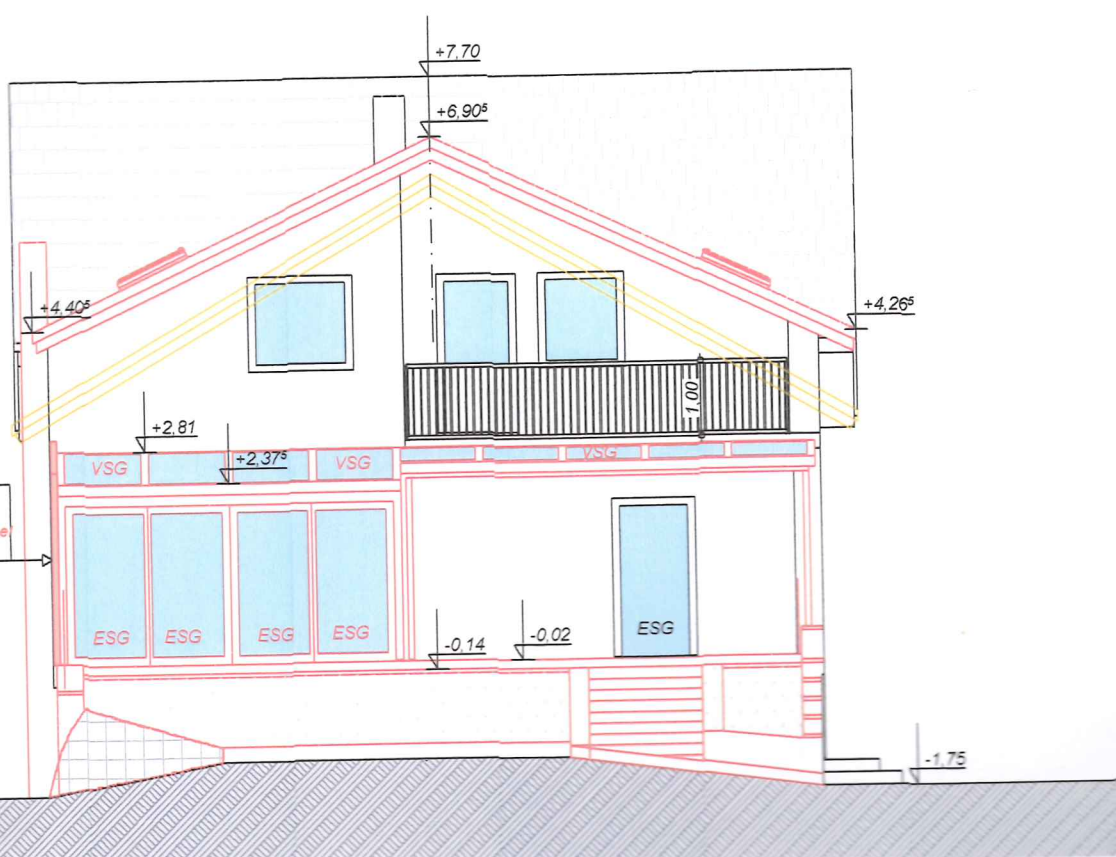
Westansicht
