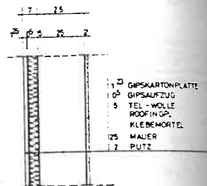
VORSATZSCHALE M=1:10
