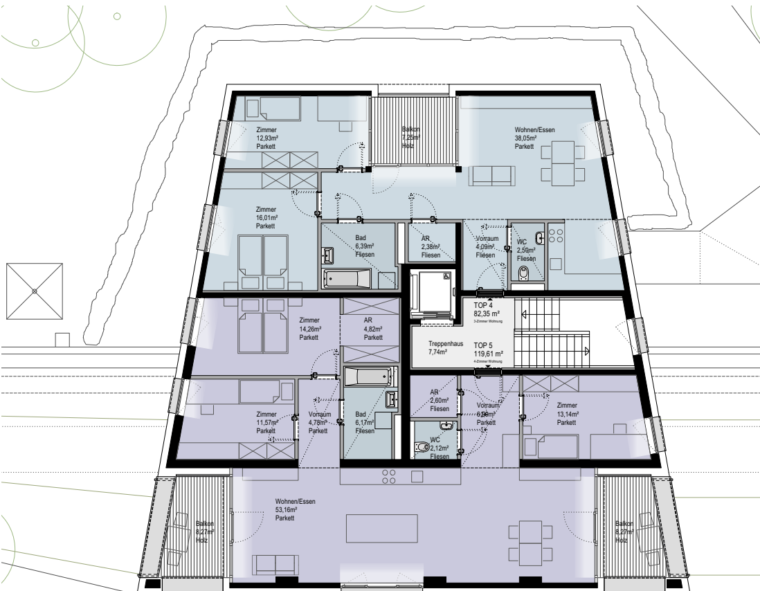
Übersichtsplan Haus 3, Ebene 02
