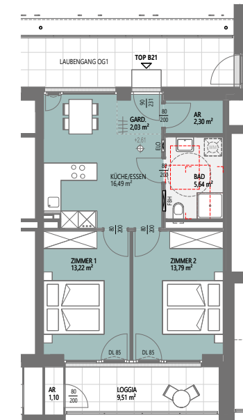
Haus B, 1.OG, Top B21 3-Zimmer-Wohnung, Wnfl. 53,47 m 2
