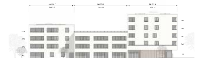
Ansicht WEST
