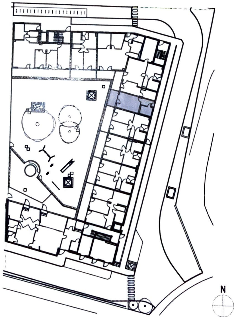
Erdgeschoss Übersicht M 1:500
