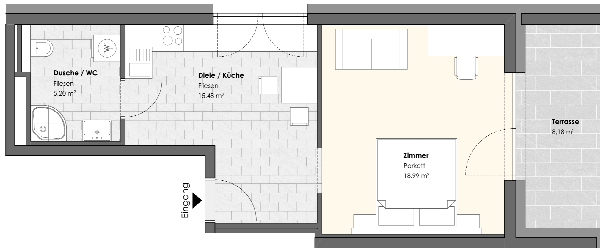
Übersicht 1.Oberirdische Geschoss M = 1 : 500
