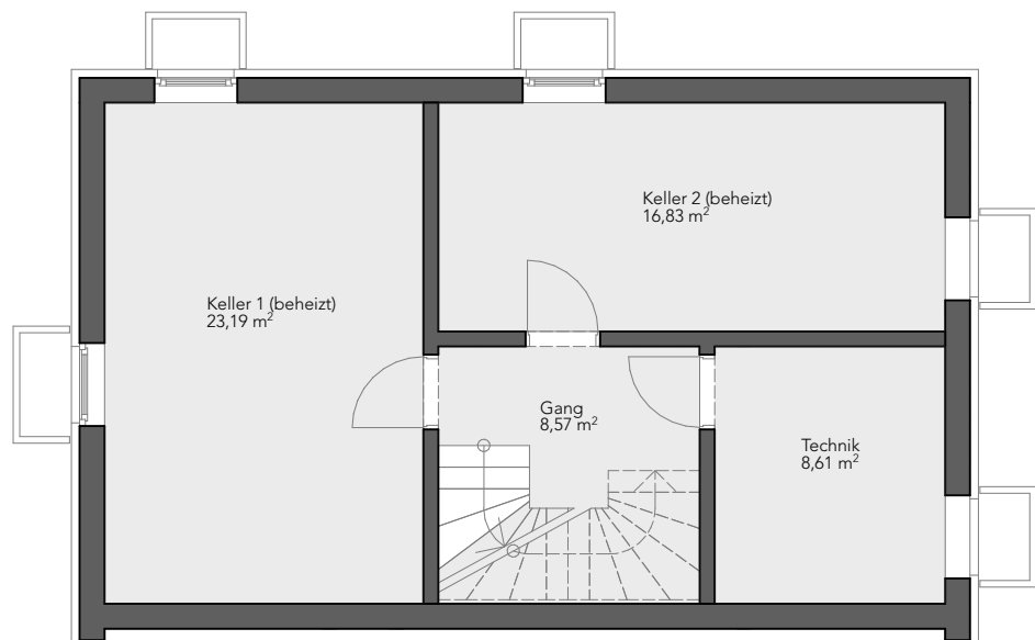
GRUNDRISS KELLERGESCHOSS
