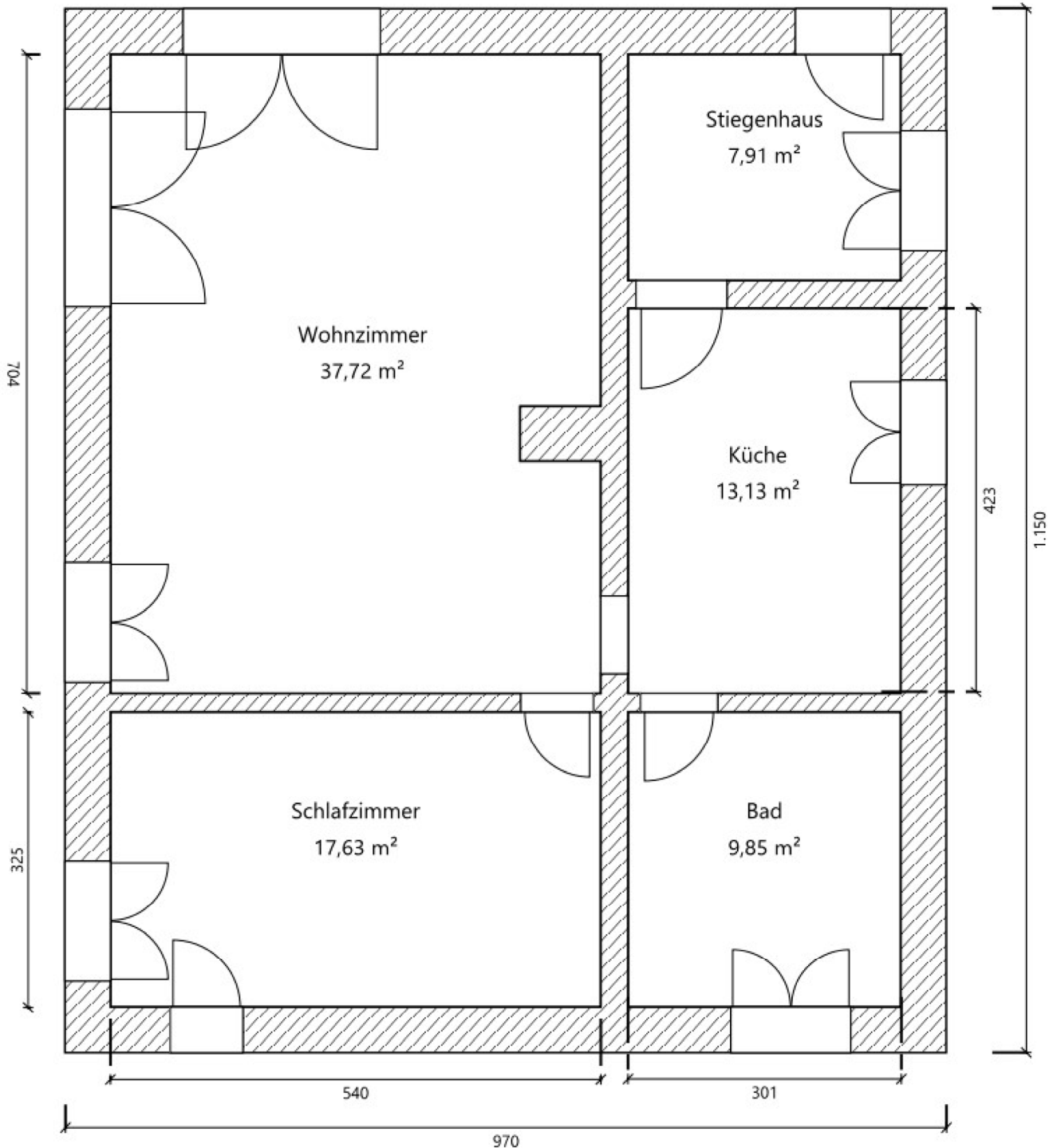
Erdgeschoss
