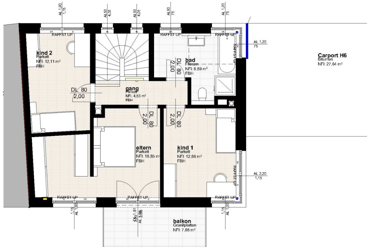
1. Obergeschoss 1:100
