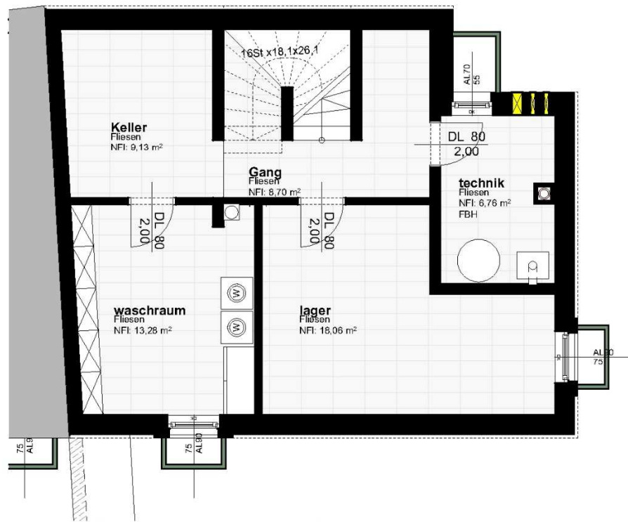
Kellergeschoss 1:100
