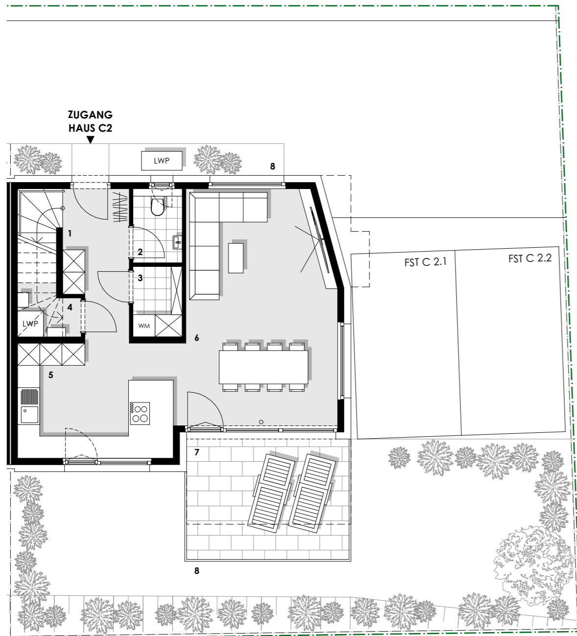
ERDGESCHOSS
